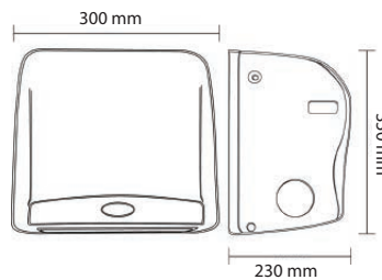
HD/58 Mini Towel Manual Dispenser
